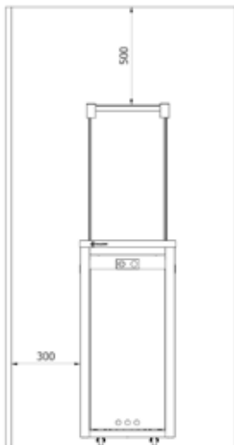
Rys. Minimalna wolna przestrzeń od materiałów/przedmiotów łatwopalnych
