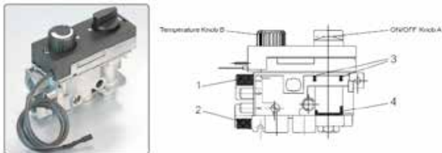
Rys. 9. Schemat sterownika GV32
