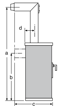
Maß a und c: mit Original-Winkelrohr dimension a and c: with original angle pipe Côtés a et c : avec conduit coude d'origine Wymiary a i c : z oryginalna rura pod kątem 90°
