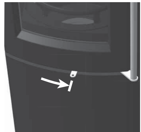
Abb. 4.18 Verbrennungslufthebel ganz rechts, Anheizstellung
