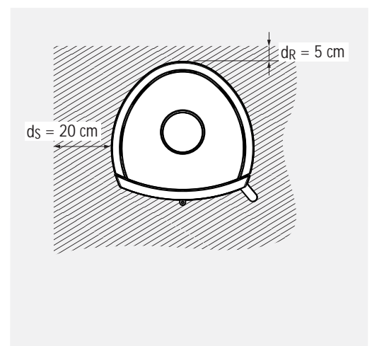
Abb. 2.4 Mindestabstände zu brennbaren Baustoffen oder Bauteilen bei DELTA plus (ohne Wassertechnik)
