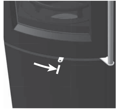
Abb. 4.9 Verbrennungslufthebel ganz rechts, Anheizstellung
