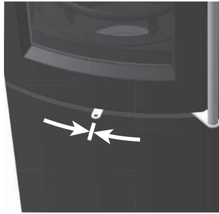
Abb. 4.8 Verbrennungslufthebel mittig, Verbrennungsluft offen, Nennwärmeleistung
