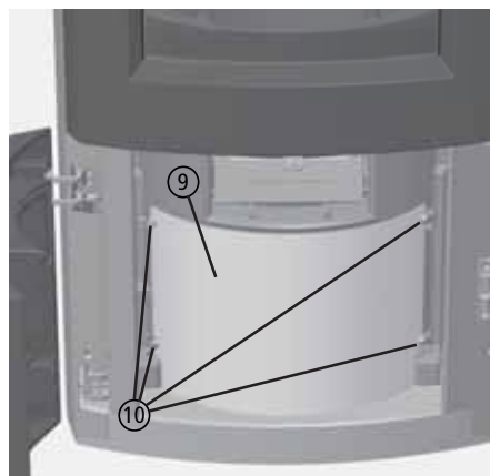
Abb. 4.25 DELTA mit LEDATRONIC: Edelstahlabdeckung vor der motorischen Luftklappe
