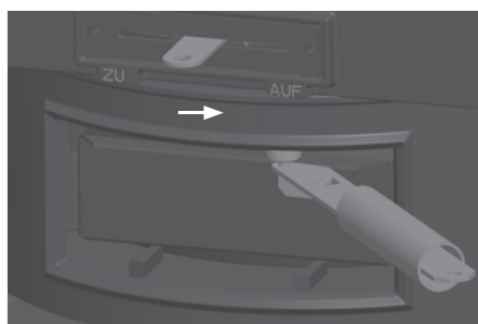
Abb. 4.5 Rüttelrost offen für Betrieb mit Unterluft
