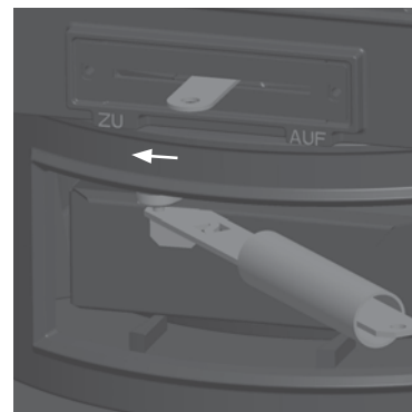
Abb. 4.11 Rüttelrost: Hebel links – Rost geschlossen
