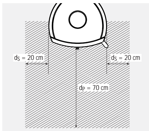
Abb. 2.2 DELTA plus: Mindestabstände im Strahlungsbereich der Sichtscheibe / im Bereich der Front
