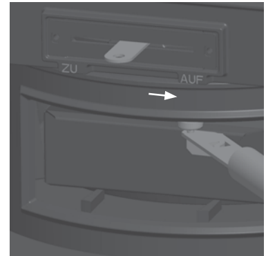
Abb. 4.17 Rüttelrost: Hebel rechts – Rost und Unterluft geöffnet
