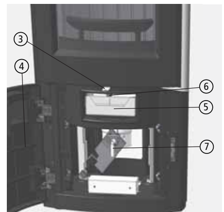
Abb. 4.2 Bedienelemente, Aschefach
