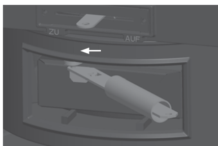
Abb. 4.4 Rüttelrost geschlossen für Betrieb mit geschlossenem Brennraumboden ohne Unterluft
