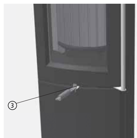
Abb. 4.6 Verbrennungslufthebel (hier mit Bediengriff)
