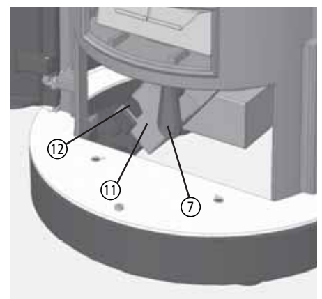
Abb. 4.26 DELTA mit LEDATRONIC: manueller Stellhebel der motorischen Luftklappe
