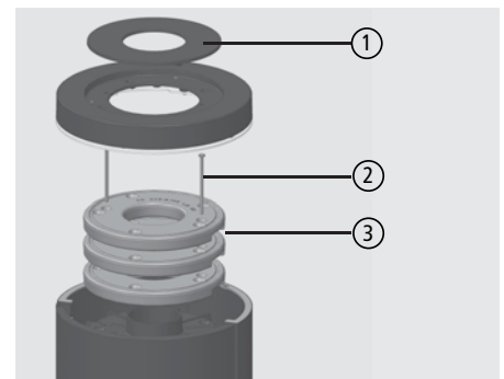
Abb. 2.1 Guss-Speichereinlagen demontieren
