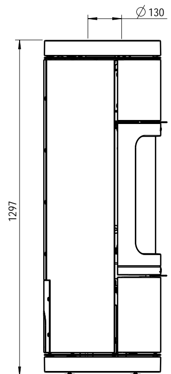
Abb. 4.13 Abgasanschluss, Maße – NOVIA W
