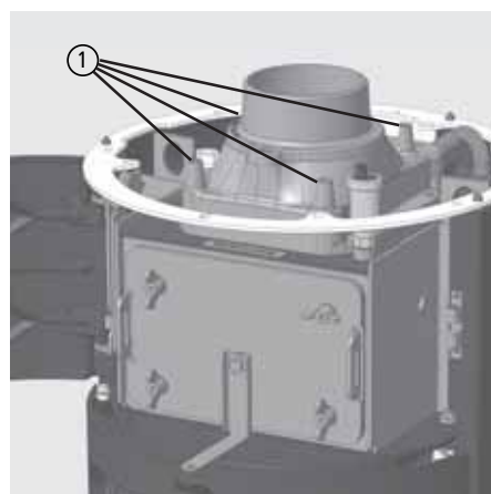
Abb. 2.24 Auflagepunkte der Deckplatte
