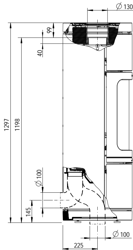
Abb. 4.12 Abgasanschluss, Maße – NOVIA plus
