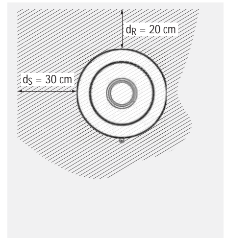
Abb. 4.2 NOVIA W: Mindestabstände zu brennbaren Materialien
