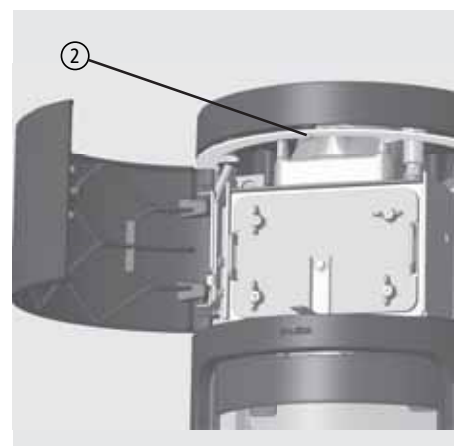
Abb. 2.25 NOVIA W: Verschraubung der Deckplatte
