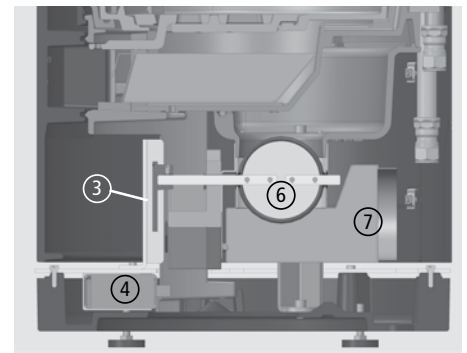
Abb. 3.3 Komponenten der LEDATRONIC im eingebauten Zustand (Beispiel NOVIA W).
