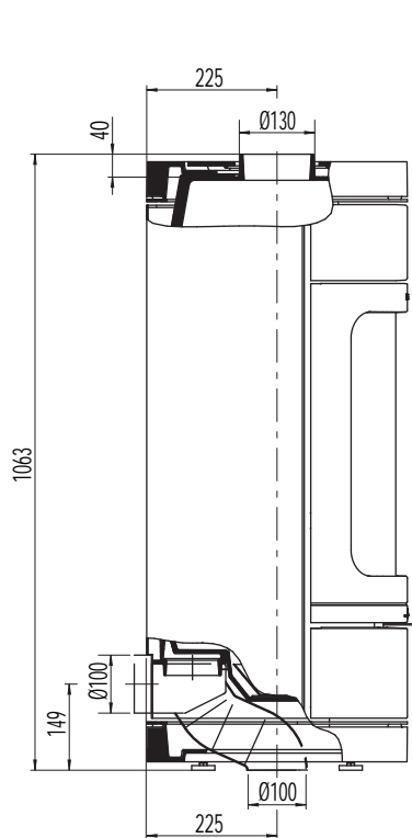
Abb. 4.10 Abgasanschluss, Maße – NOVIA C
