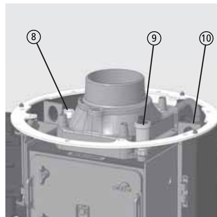
Abb. 2.21 NOVIA W: Gewindemuffen für automatischen Entlüfter, TAS- und Kesselfühler
