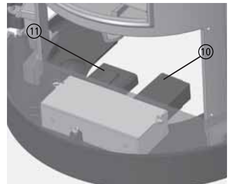
Abb. 2.17 Steuerung und Batteriegehäuse, elektronische Heizhilfe
