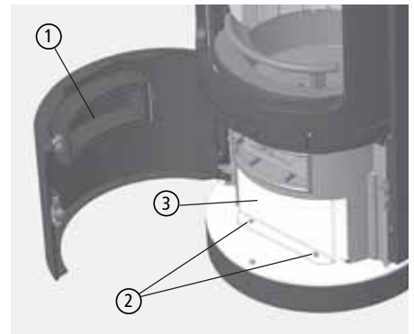
Abb. 2.11 senkrechte Zierringblende (Edelstahlabdeckung) entnehmen
