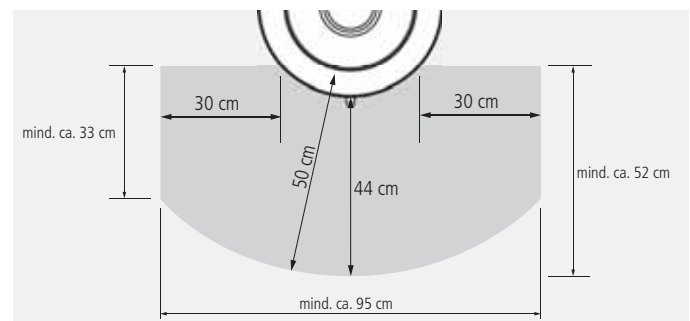
Abb. 4.8 Nicht brennbarer Belag vor der Feuerraumöffnung
