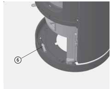
Abb. 2.15 eingetragenes LED-Element
