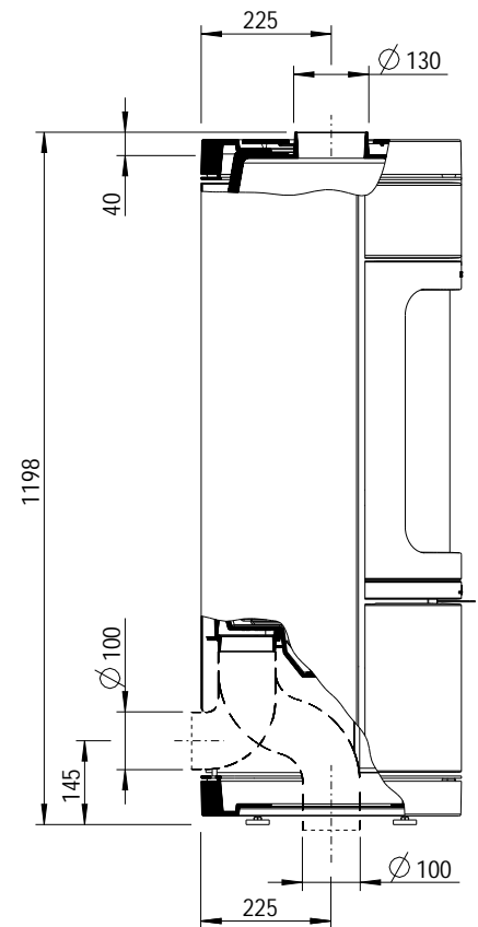
Abb. 4.11 Abgasanschluss, Maße – NOVIA CL
