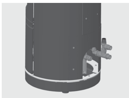
Abb. 2.23 NOVIA W: fertig montierter Anschlussatz
