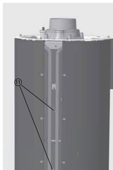
Abb. 2.22 NOVIA W: Kabelklammern
