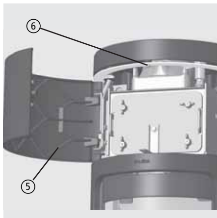
Abb. 2.20 NOVIA W: Revisionstür und Verschraubung der Deckplatte
