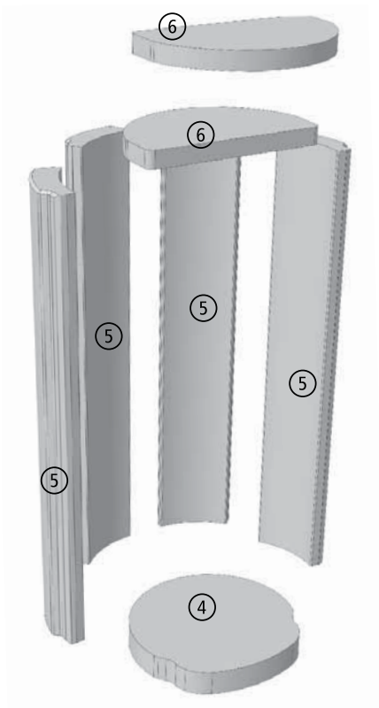
Abb. 5.1 Ersatzteilübersicht für PEPPA / PEPPA tec- Feuerraumauskleidung
