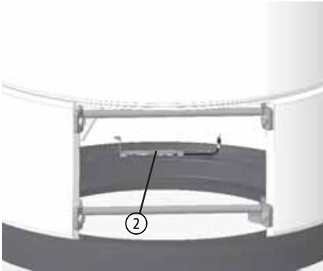
Abb. 3.17 LED-Element, elektronische Heizhilfe
