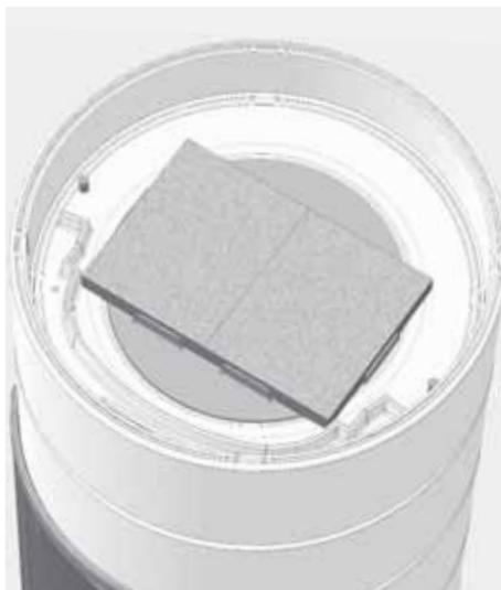
Abb. 3.4 Lage der Katalysatorplatten beim PEPPA tec, Blick von oben bei abgenommener Deckplatte
