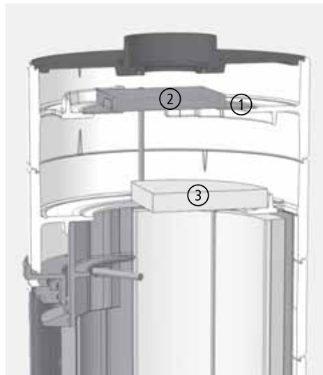
Abb. 3.20 Lage der Katalysator-Elemente beim PEPPA tec, Schnittdarstellung
