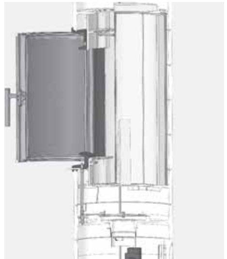
Abb. 4.32 Aufrichten des Bodensteins im Brennraum
