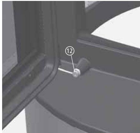
Abb. 3.15 gespannte Türfeder
