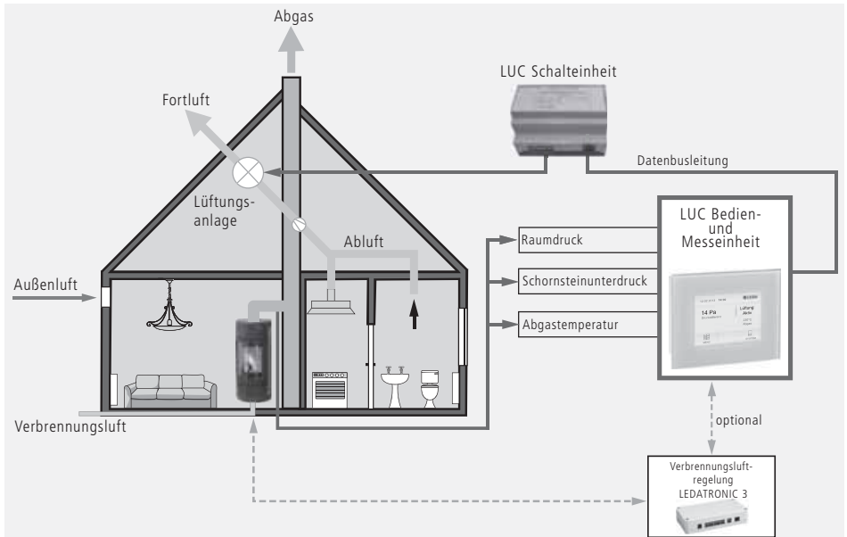
Abb. 3.1 Systemdarstellung, Feuerstätte, Lüftungsanlage, optional LT3 zusammen mit LUC
