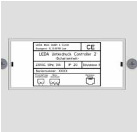
Abb. 10.1 Gerätekenzeichnung auf der Schalteinheit des LUC
